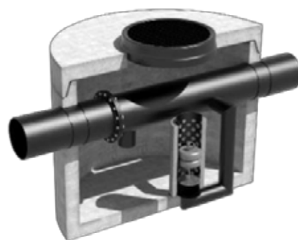
Koalescensavskiljare med by-pass ESK-B
