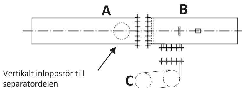
Fig.1.5 Element av ESK-B II / ESK-BH II-Avskiljarutrustning
